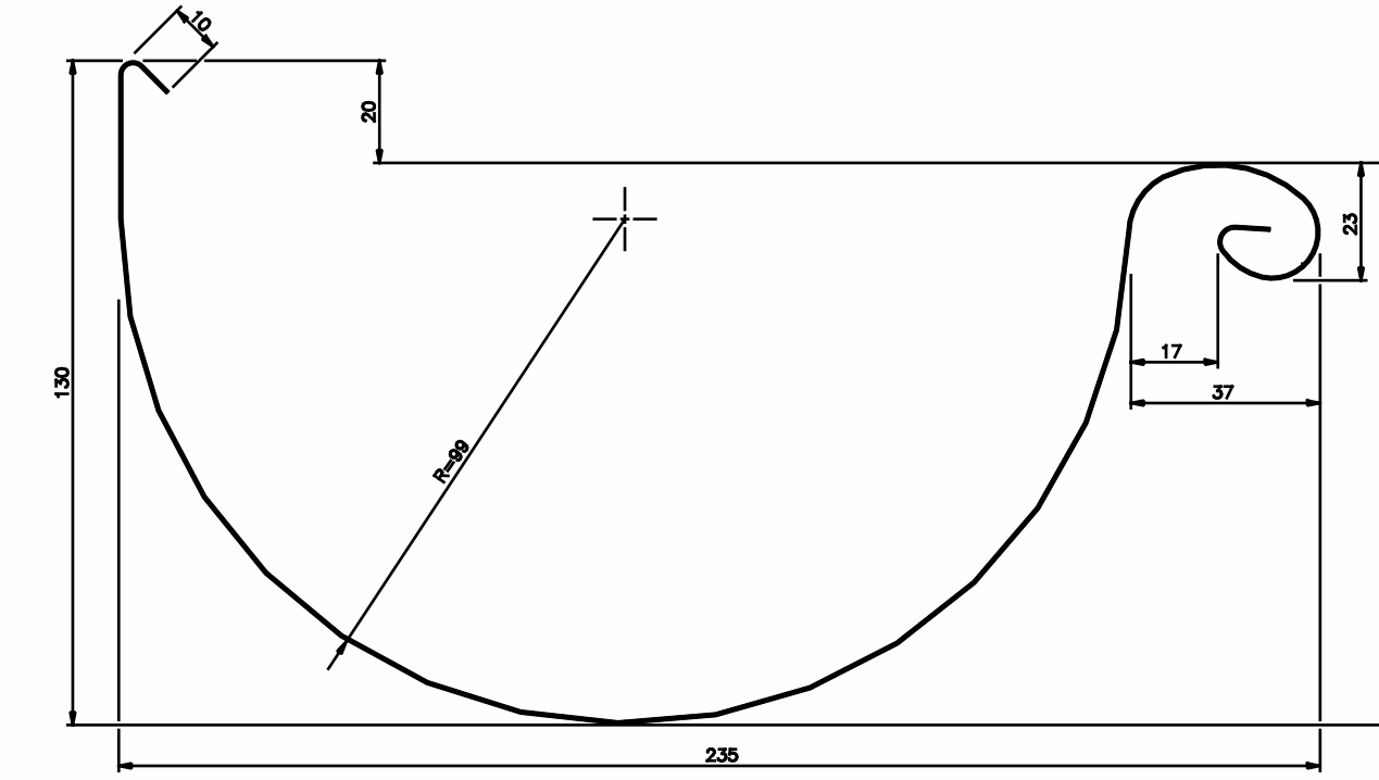
MASTGOOT M44 Materiaal: NedZink NTZ
