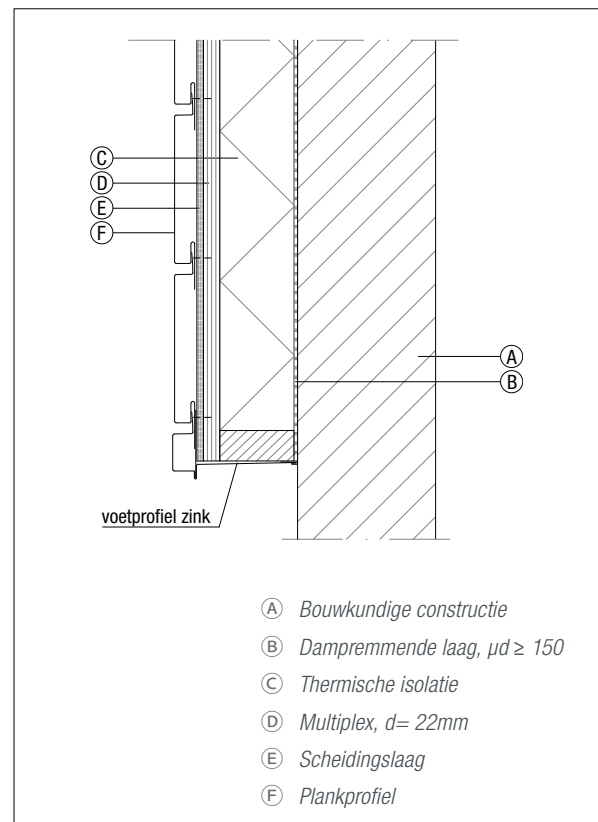
Figuur 6.4.28 Onder aansluiting
