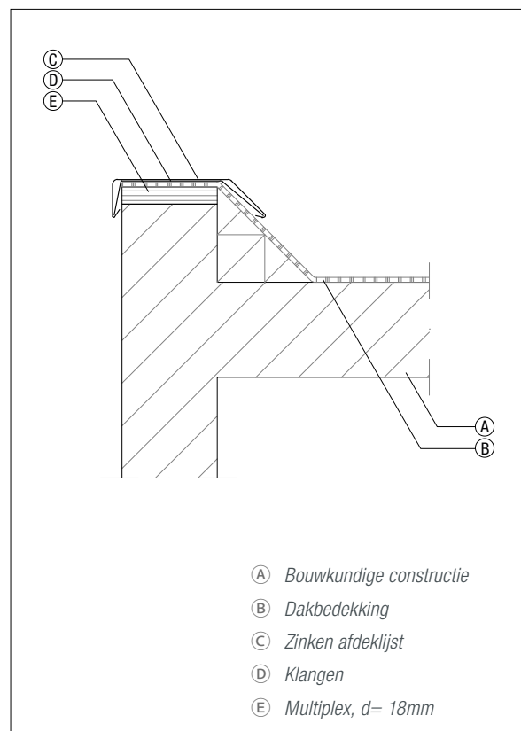
Figuur 7.1.2 Zinken deklijst met platte band
