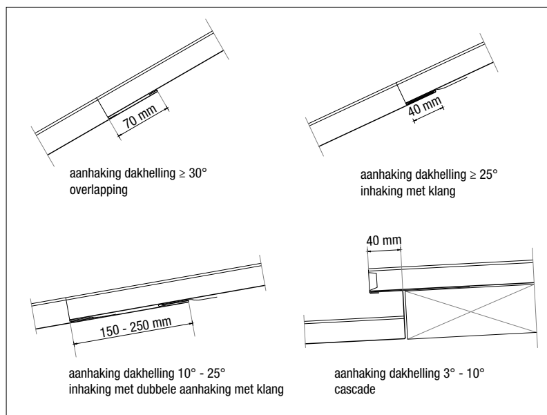
Figuur 5.2.3 Dwaarsverbinding dakhelling
