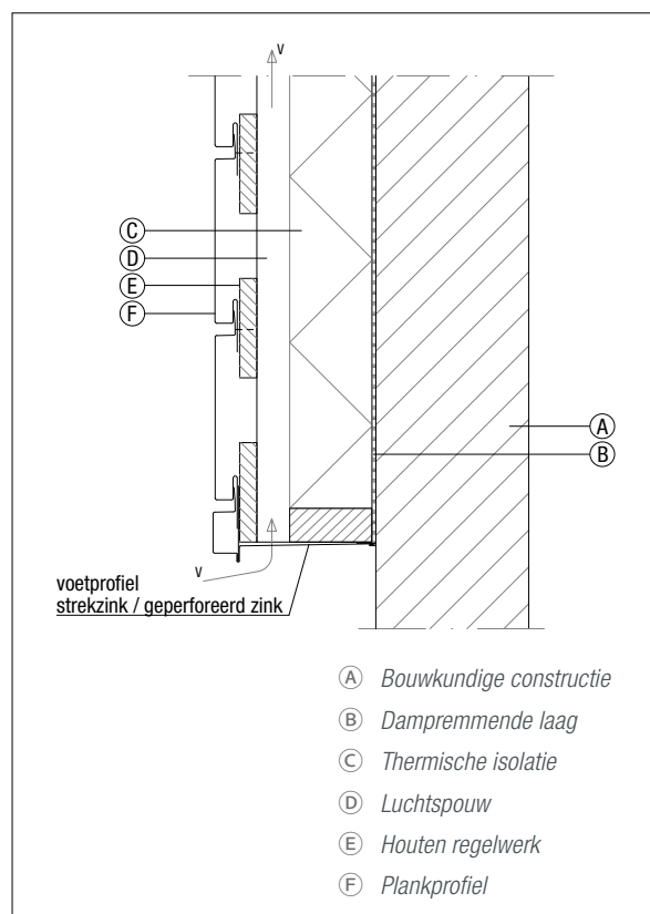
Figuur 6.4.13 Onder aansluiting
