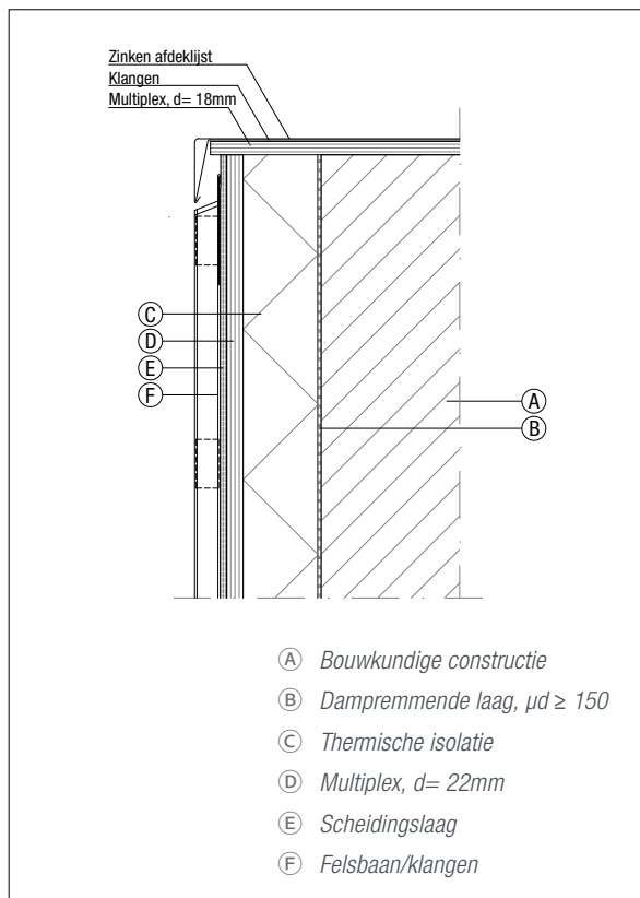
Figuur 6.1.21 Bovenaansluiting dakrand
