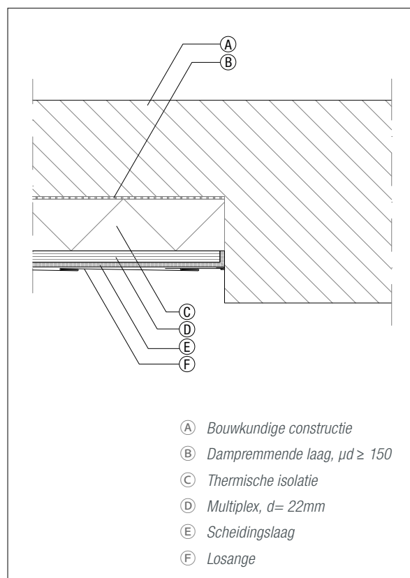
Figuur 6.3.21 Aansluiting muur
