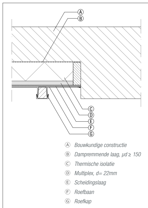
Figuur 6.2.27 Aansluiting muur
