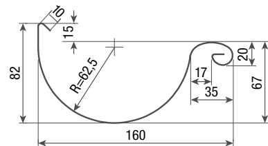
Mastgoot M30 materiaal NedZink NTZ
