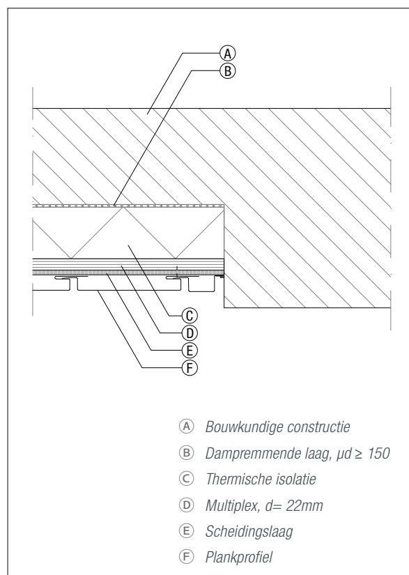
Figuur 6.4.25 Aansluiting muur
