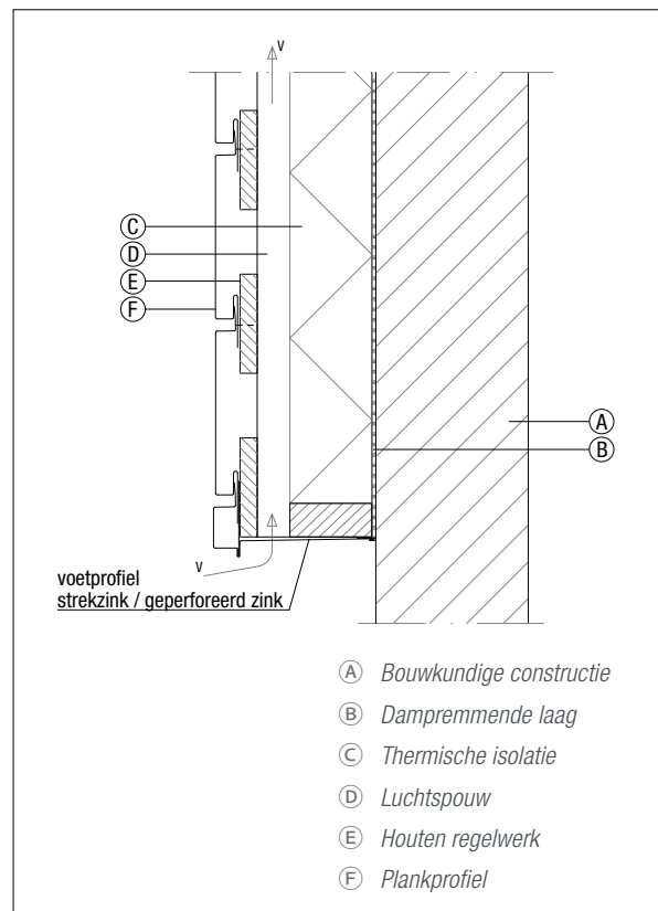
Figuur 6.4.13 Onder aansluiting
