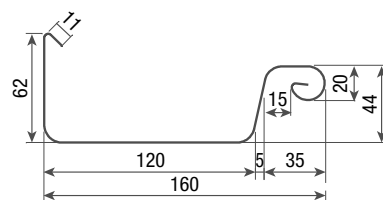
Bakgoot B30 materiaal NedZink NTZ
