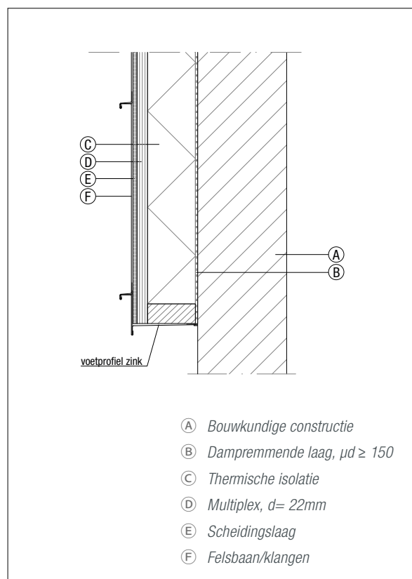
Figuur 6.1.29 Onderaansluiting
