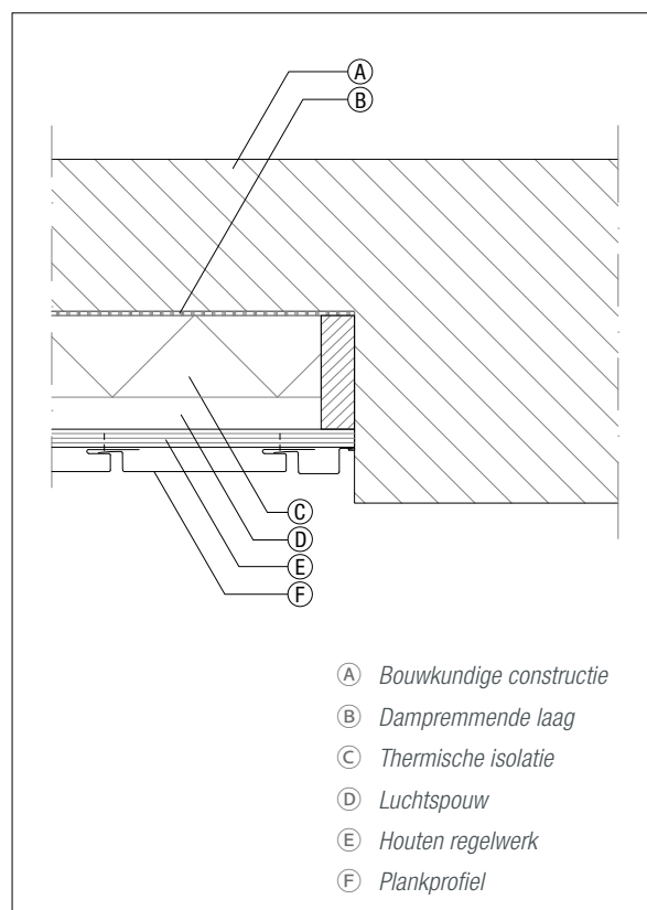
Figuur 6.4.10 Aansluiting muur
