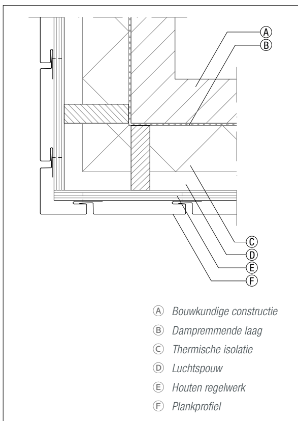
Figuur 6.4.11 Buitenhoek
