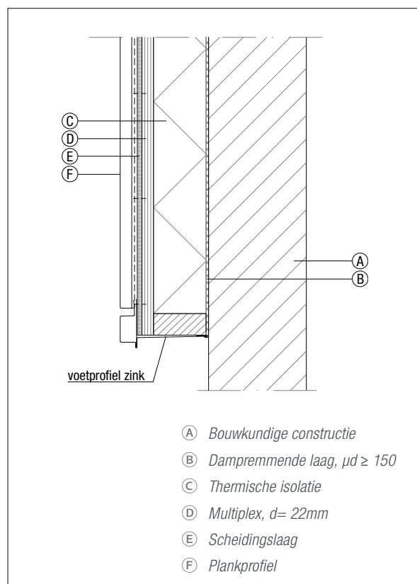
Figuur 6.4.21 Onderaansluiting
