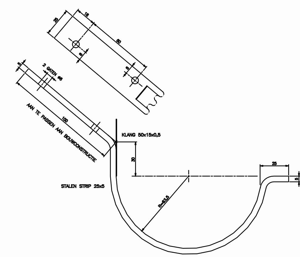
BEUGEL VOOR MASTDOOT M30 WISPAAL THERRSCH VERBODT DEN 1270
