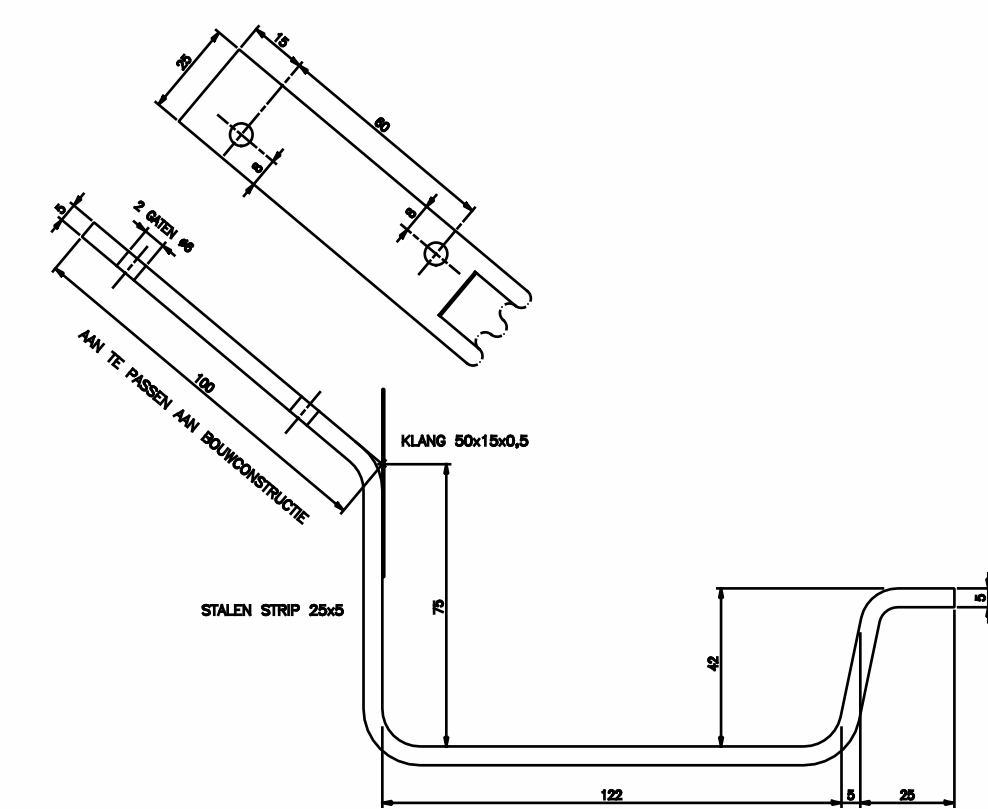
BEUGEL VOOR BANKDOOT B30 WISPAAL THERRSCH VERBODT DEN 1270
