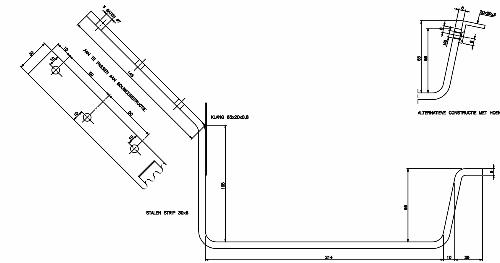
BEUGEL VOOR BANKDOOT B44 WISPAAL THERRSCH VERBODT DEN 1270
