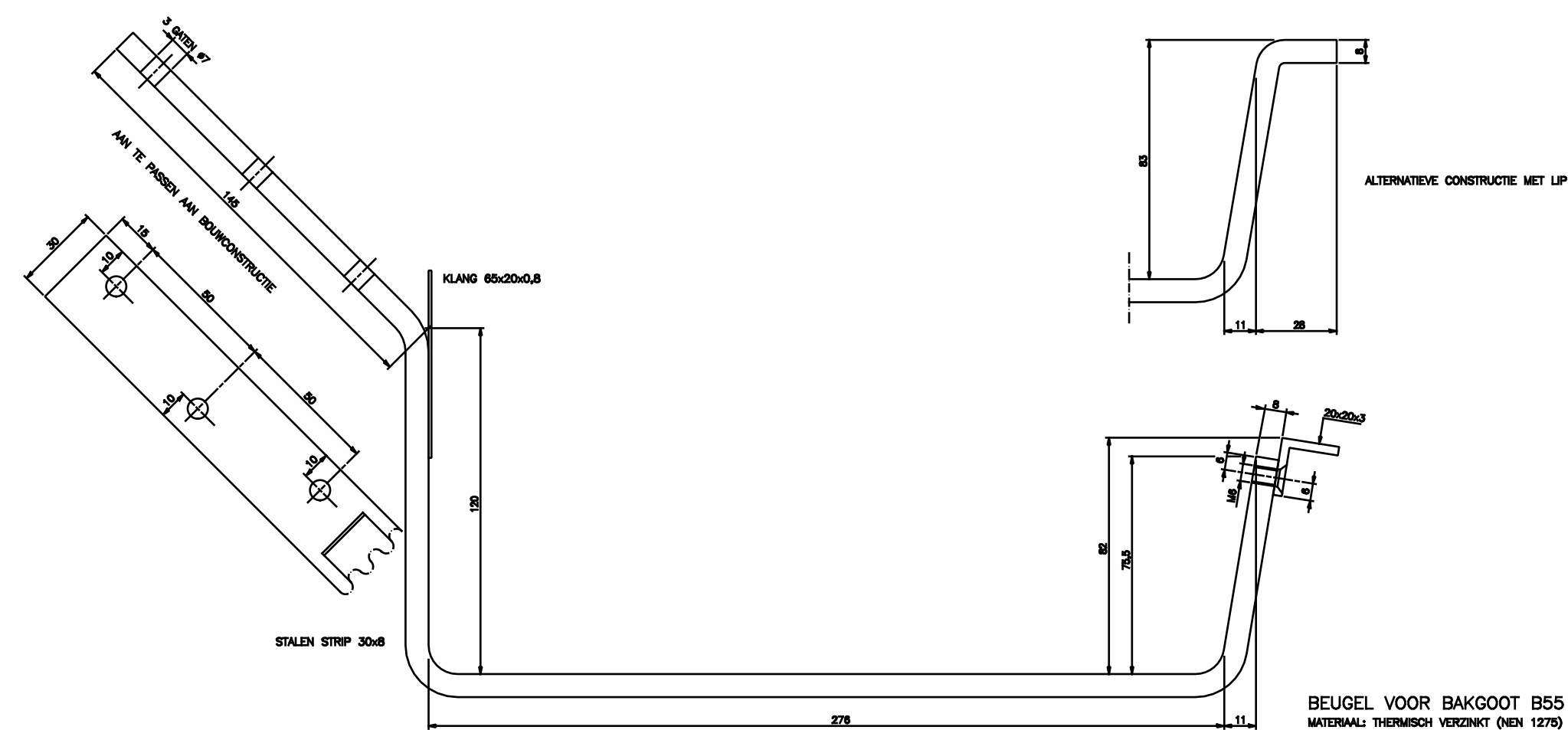
BEUGEL VOOR BANKDOOT B55 WISPAAL THERRSCH VERBODT DEN 1270
