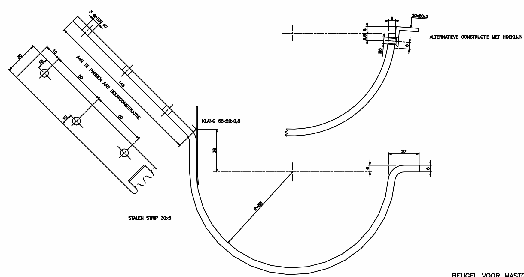
BEUGEL VOOR MASTDOOT M37 WISPAAL THERRSCH VERBODT DEN 1270
